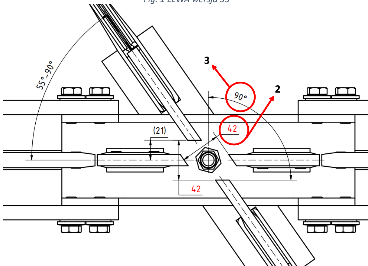
Fig 2 LEWA wersja 55°
