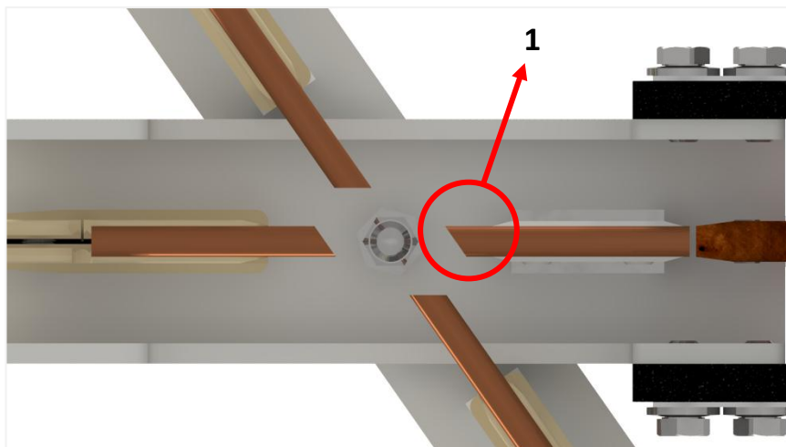
Fig. 1 LEWA wersja 55°
